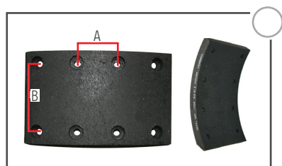
Bremsbeläge Ausführung 1
