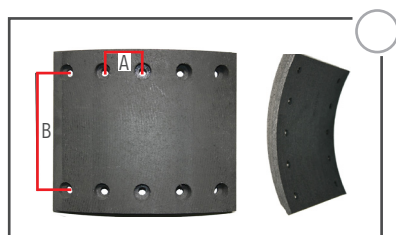
Bremsbeläge Ausführung 2
