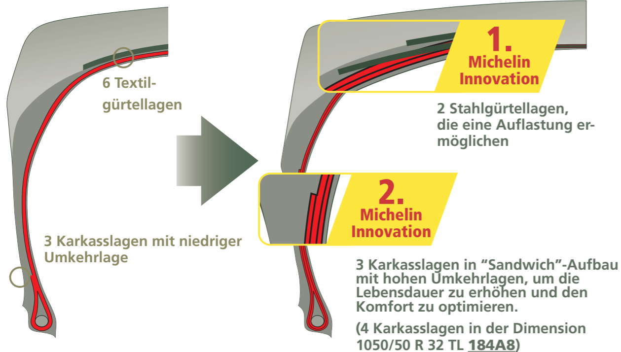
MICHELIN MegaXBib innovativer Aufbau
